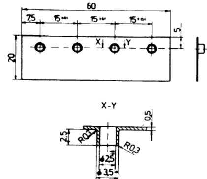
Folie mit eingespritzten Isolierbuchsen
