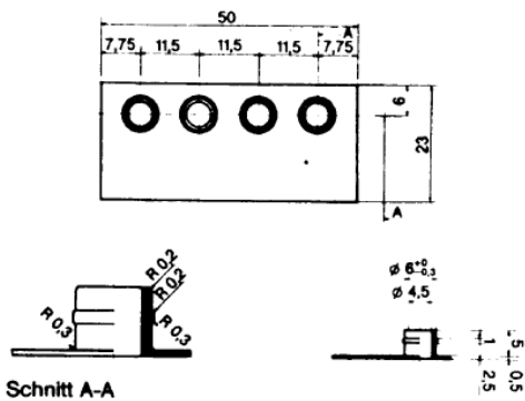
Folie mit eingespritzten Isolierbuchsen
